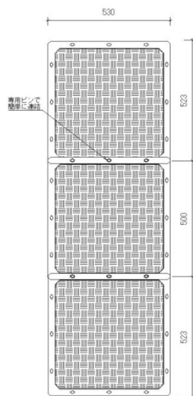
MEPトレイ-N 連結寸法
