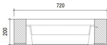
MEPトレイ-H 木枠H=200 土厚125mm
